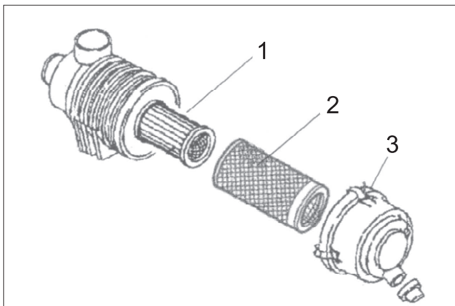
1 Ilmansuodatinpanos
