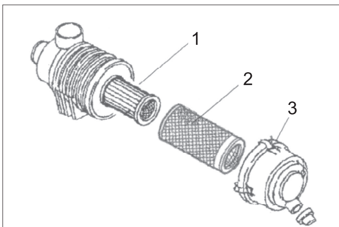
1 Luftfilterindsats
