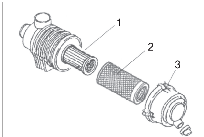
1 Gaisa filtra ieliktnis
